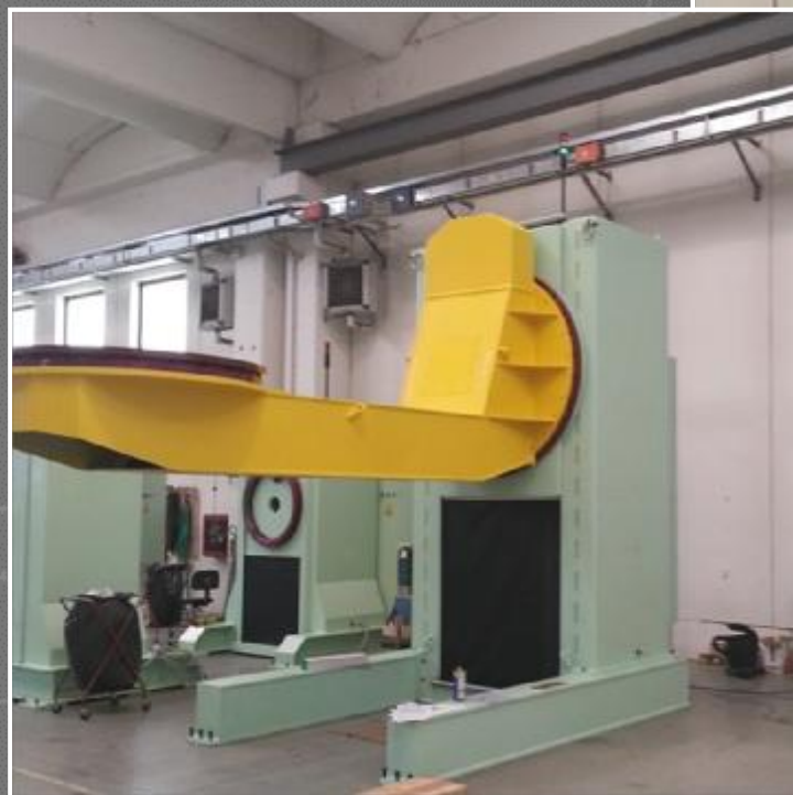
Трехосевые позиционеры для вращения рам экскаваторов
