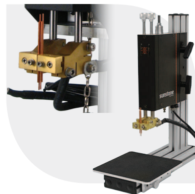
Головка с параллельными электродами
