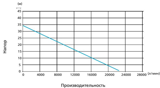
WEDA D100N
