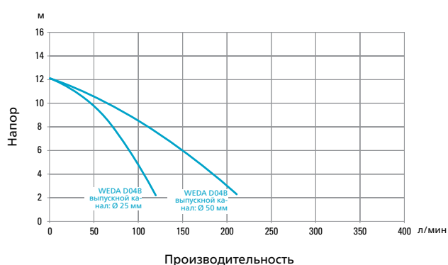
WEDA D04BN
