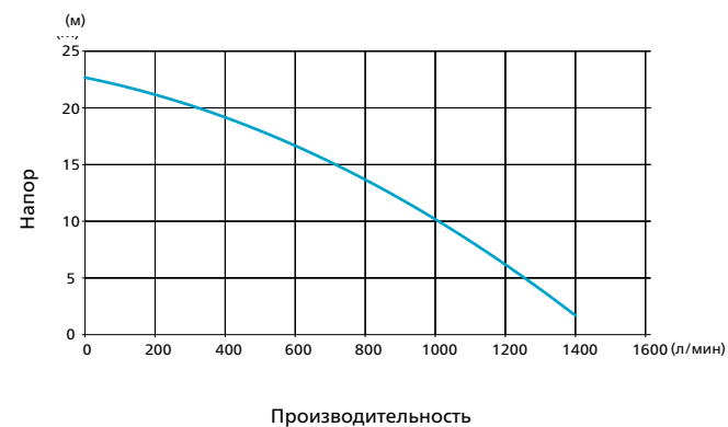
WEDA D40N
