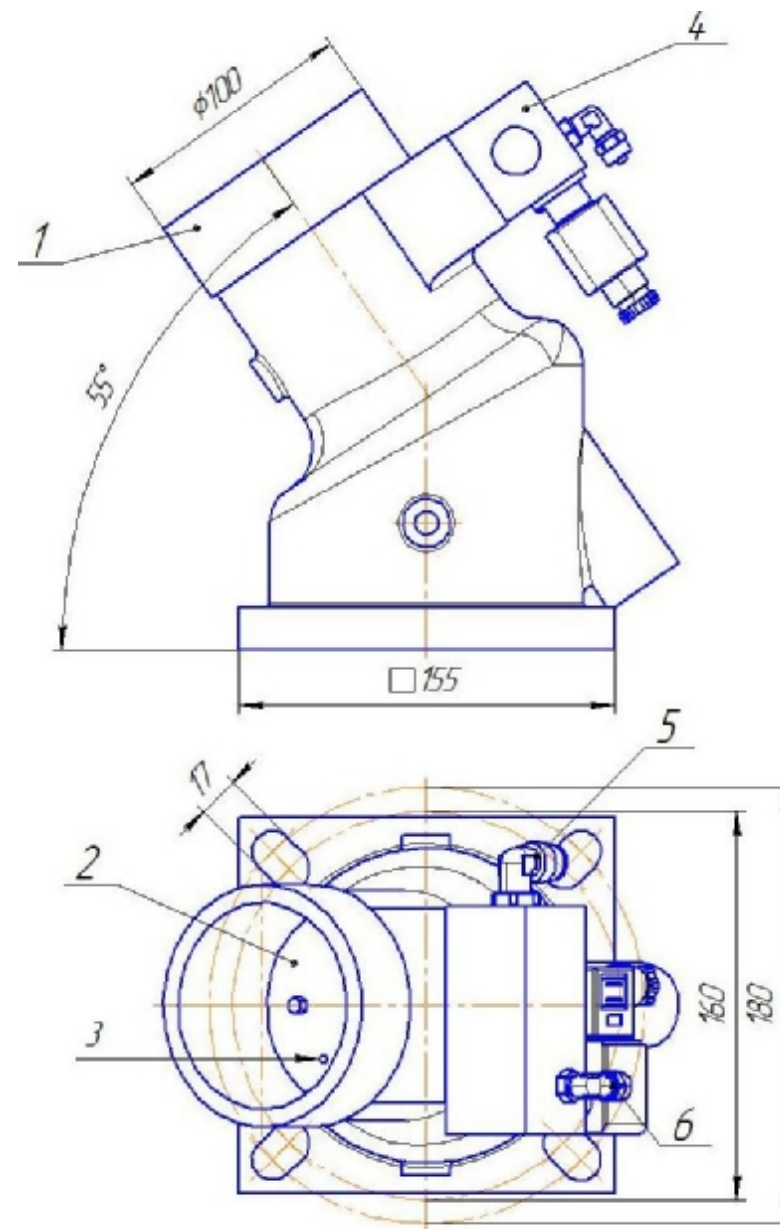
Рисунок 4. Клапан впускной.
