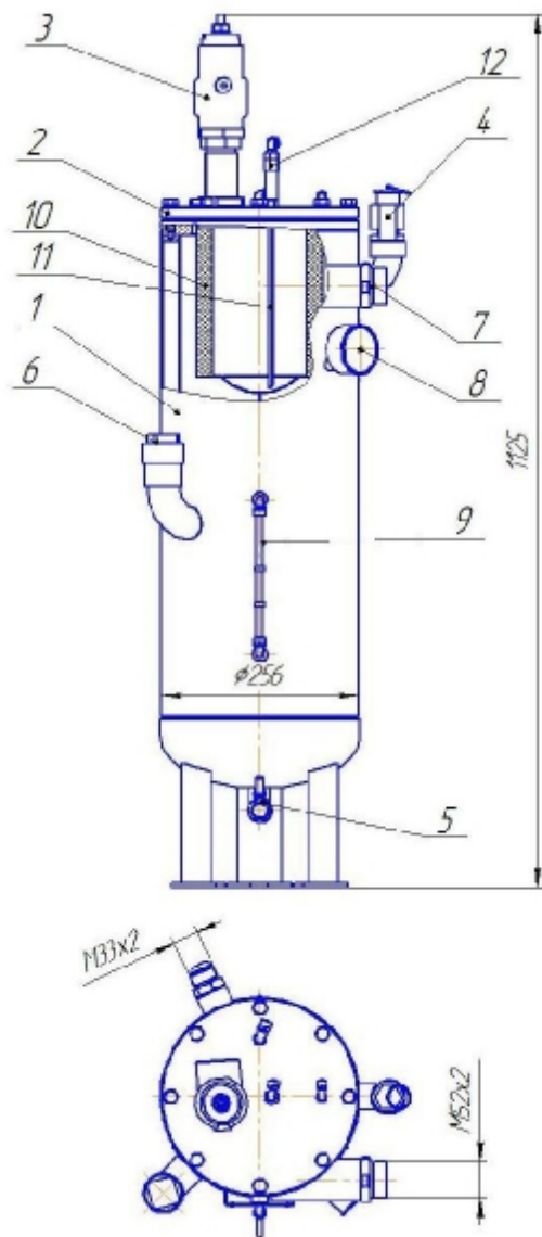
Рисунок 5. Маслоотделитель.
