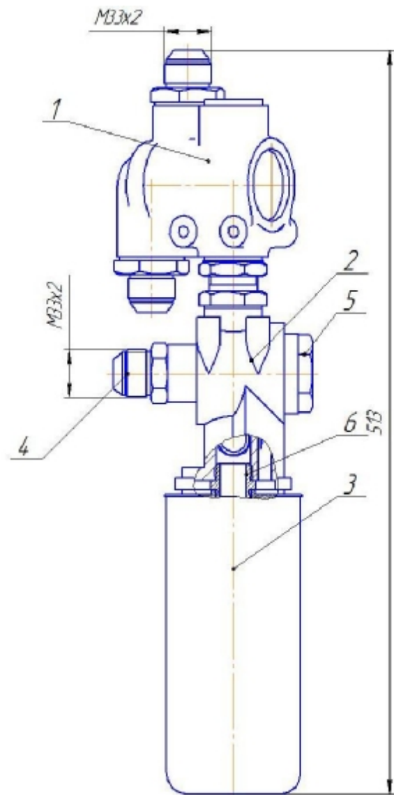
Рисунок 7. Блок распределения.
