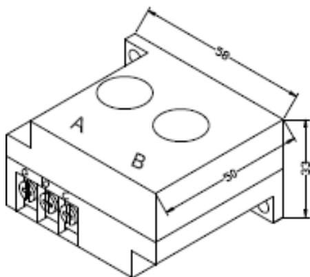
Рисунок 4.1.3. Габаритные размеры СТ2 СТ2
