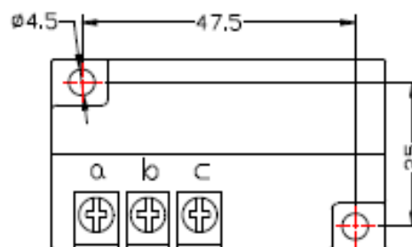
Рисунок 4.1.4. Установочные размеры
