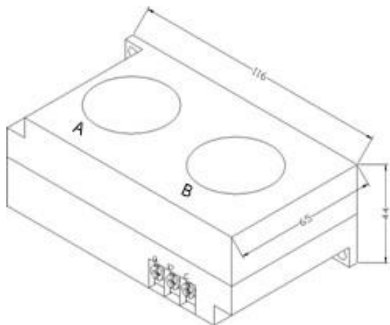
Рисунок 4.1.1. Габаритные размеры СТ1 СТ1
