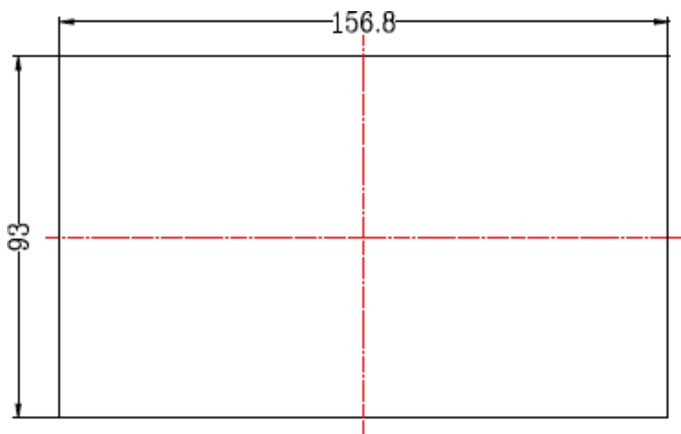
Рисунок 4.1.6 Размеры отверстий
