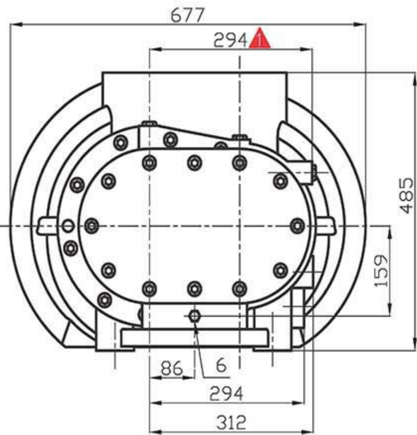
A-A(3:1)
