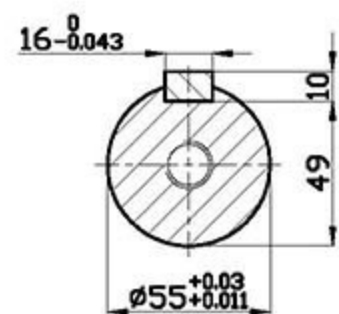
A-A(3:1)
