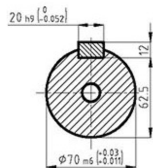
A-A(3:1)
