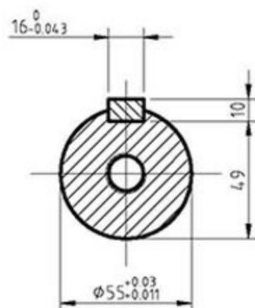
A-A(3:1)
