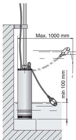
3.83.00703 Модификация с поплавковым выключателем
