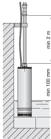
5.93.00072 Ausführung ohne Schwimmerschalter
