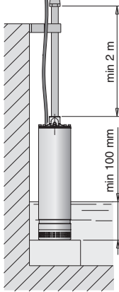
Οδηγίες για χρήση χωρίς φλοτέρ
