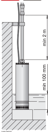
Ejecución sin interruptor de nivel
