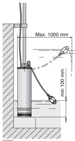
Ejecución con interruptor de nivel
