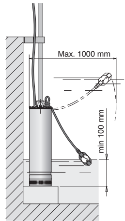
5.93.00072 Ausführung mit Schwimmerschalter
