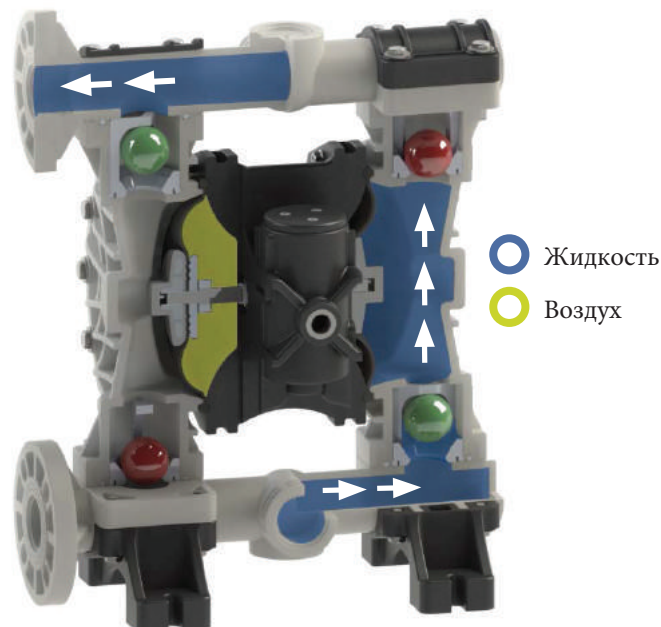
2. Цикл «Нагнетание»
