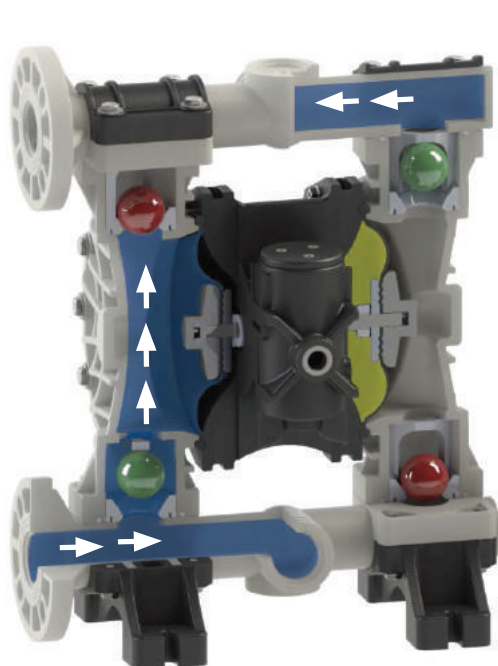
1. Цикл «Всасывание»
