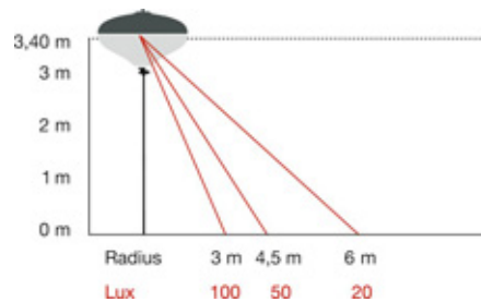
Освещение с помощью галогенной лампы на треноге высотой 3,4 метра
