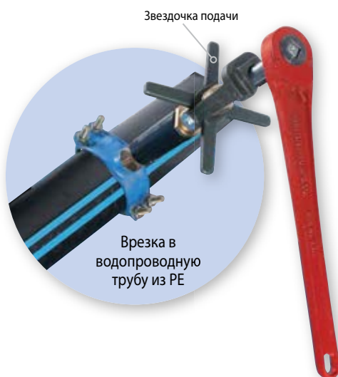
Звездочка подачи
