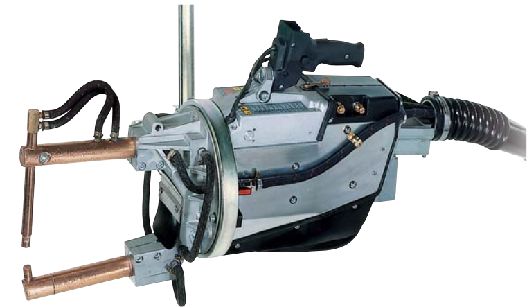
Клещи 3321 с блоком ТЕ300
