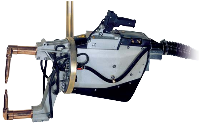
Клещи 3328 с блоком ТЕ300
