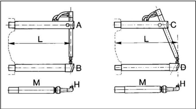
Характеристики плеч для клещей 3322
