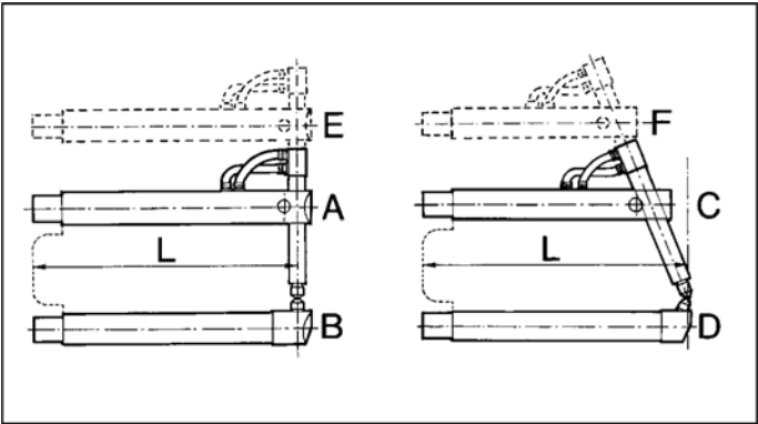
ПЛЕЧИ ДЛЯ КЛЕЩЕЙ 3327—3328
