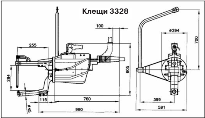
ПЛЕЧИ ДЛЯ КЛЕЩЕЙ 3327—3328
