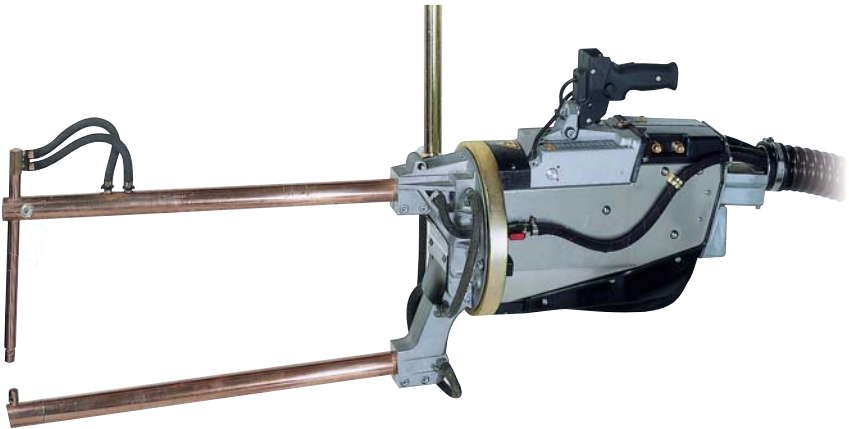
Клещи 3324 с блоком ТЕ300
